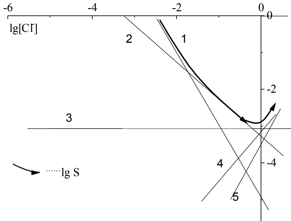
Рис. 2.2. Концентраційно-логіфімічна діаграма для системи: осад \text{PbCl}_2 — іони \text{Cl}^- в розчині
