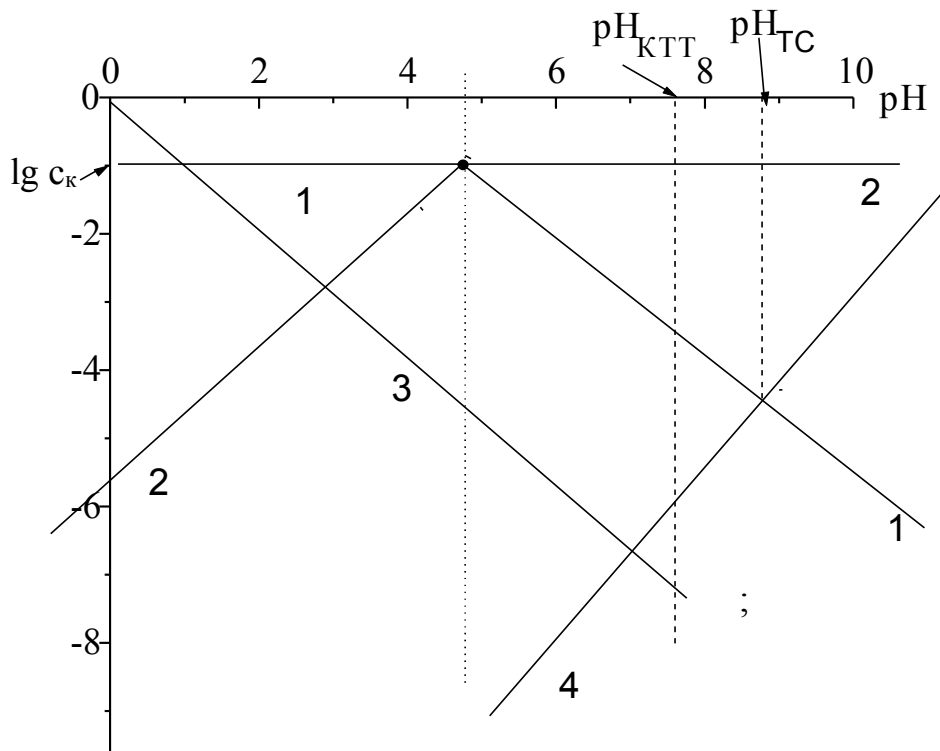
Рис. 6.1. Концентраційно-логіфічна діаграма для системи слабка кислота НА – супряжена основа А
